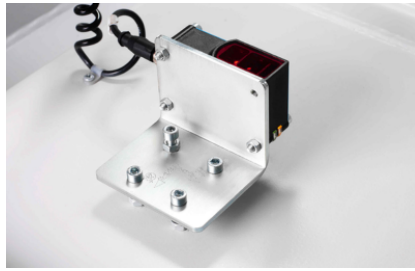
HSM TCS (TorsionControlSystem) voor kantelbewaking van de persplaat
