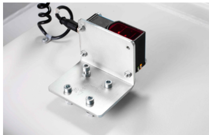
TCS (TorsionControlSystem) voor kantelbewaking van de persplaat
