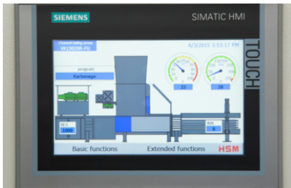
Controle van het persproces via fotocel
