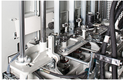
Legatura verticale
