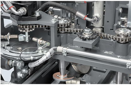
Legatura verticale delle balle con filo metallico
