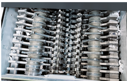
1° livello pretriturazione con sistema a quattro alberi, composto da due alberi da caricamento e due alberi da taglio.
