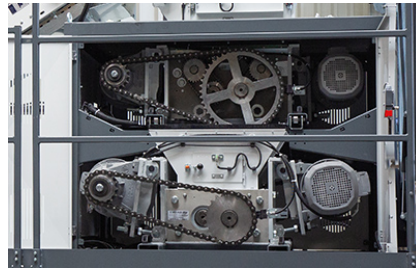
Impianto di smaltimento di documenti a due livelli completamente automatico.
