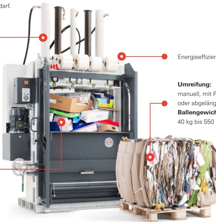
HSM V-Press 860 plus
